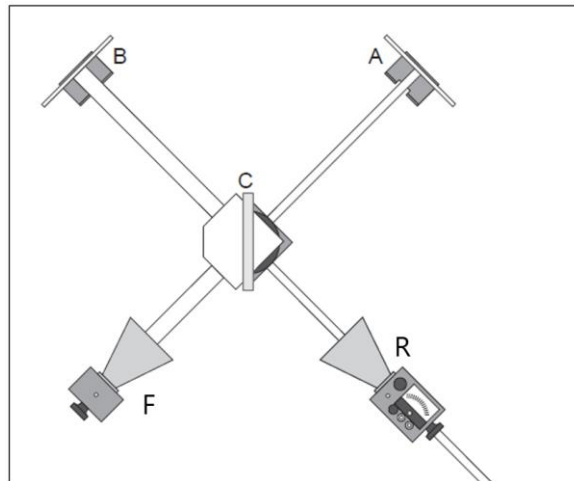
Fig. 1. Esquema del Interferómetro de Michelson empleado en la práctica.
